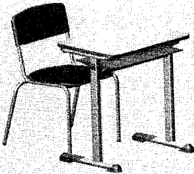
CONJUNTO ALUNO COD-343 CJA-03 ALTURA DO ALUNO 1,46 A 1,76M
