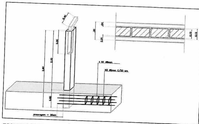
ESQUEMA DE ENGASTAÇÃO DO PILAR DE CONCRETO e VIGA BALDRAME ESC 1:25
