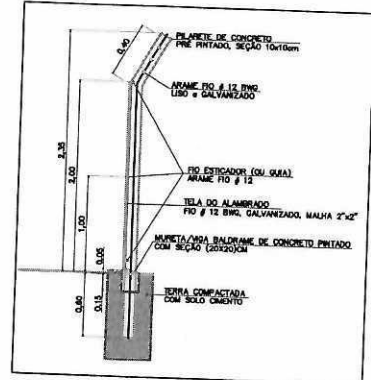
CORTE ESQUEMÁTICO DO ALAMBRADO 2 e 3 SEM ESCALA
