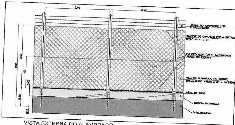
VISTA EXTERNA DO ALAMBRADO ESC 1:25
