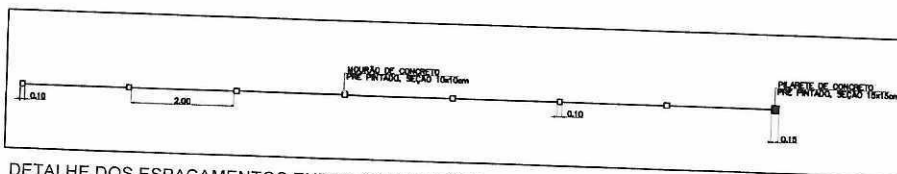
DETALHE DOS ESPAÇAMENTOS ENTRE OS MOURÕES DE CONCRETO E DO PILARETE DE CONCRETO ESC 1:50
