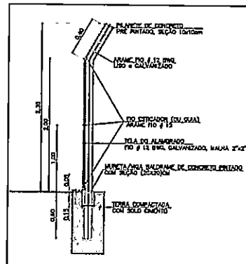
CORTE ESQUEMÁTICO DO ALAMBRADO 2 e 3 SEM ESCALA
