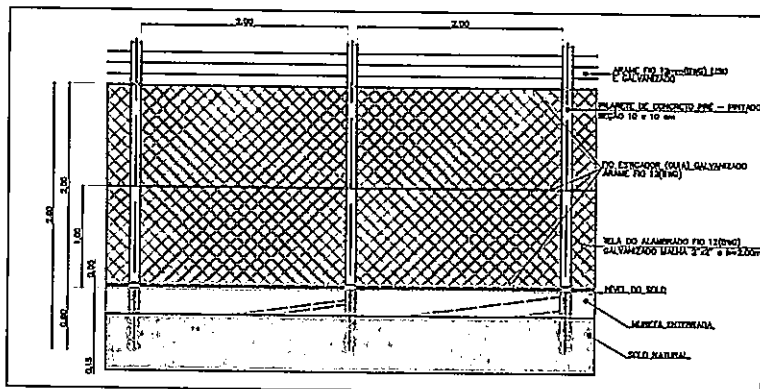
VISTA EXTERNA DO ALAMBRADO ECO 123
