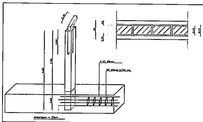
ESQUEMA DE ENGASTAÇÃO DO PILAR DE CONCRETO e VIGA BALDRAME ECO 123
